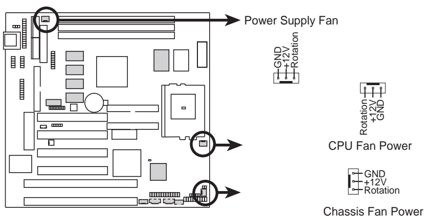
P5S-B 12Volt Cooling Fan Power
