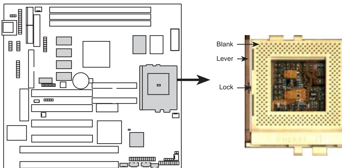
P5S-B ZIF Socket 7
