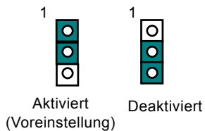
JP2 (Lautsprecher)
