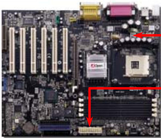
4-Pin 12V ATX-Netzanschluss
