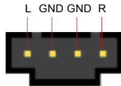
CD-IN-Anschluss
