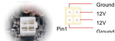
4-Pin 12V ATX 電源接頭
