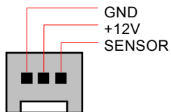
第二系統風扇電源接頭
