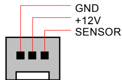
第一系統風扇電源接頭
