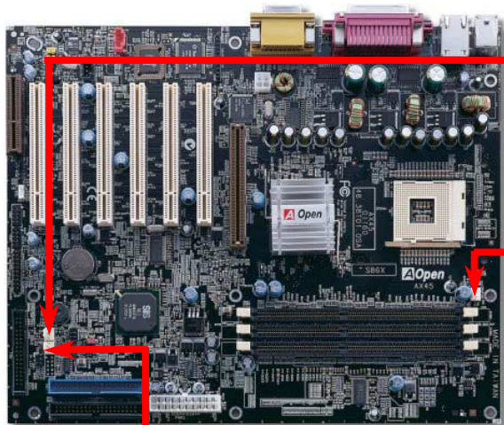
FAN3 コネクタ
