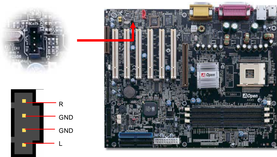
CD 入力コネクタ
